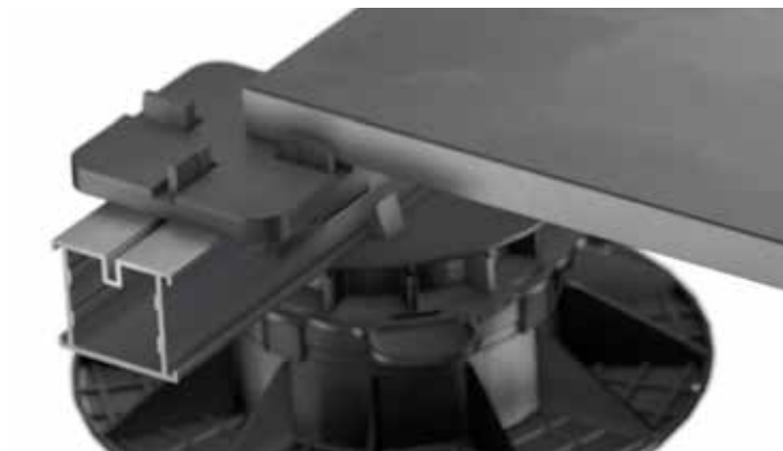
Einstellhöhen für Stelz und Plattenlager von 11 - 570 mm
